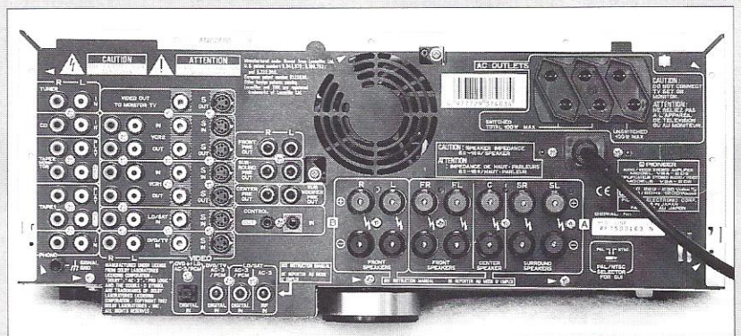
De achterzijde van de VSA-E06
